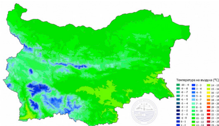
Фигура 3: Средна месечна температура на въздуха и сума на валежите в България за периода 1991 – 2020 г. по данни на НИМХ/ Източник: Изчислени са климатичните норми за България за новия референтен период 1991-2020 г. – Новини – БЪЛГАРСКА ТЕЛЕГРАФНА АГЕНЦИЯ (bta.bg) .
