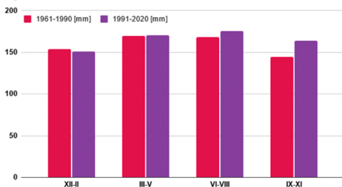
Сума на валежите по сезони
