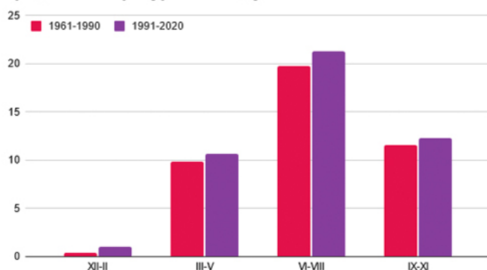
Средна температура на въздуха по сезони
