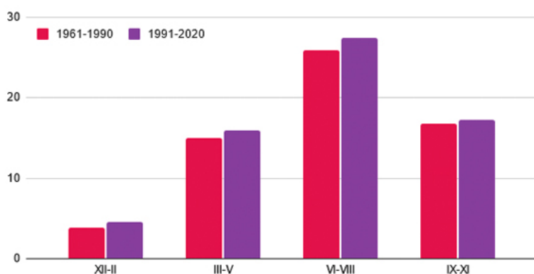
Средна от максималните стойности на температура на въздуха в България по сезони.
